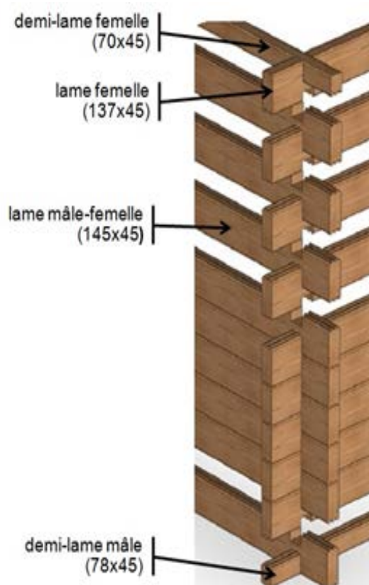
Figure 60 – Principe d'emboîtement des lames de bois
