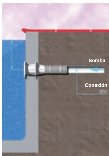
Instalación boquillas
