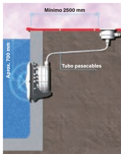
Instalación proyector
